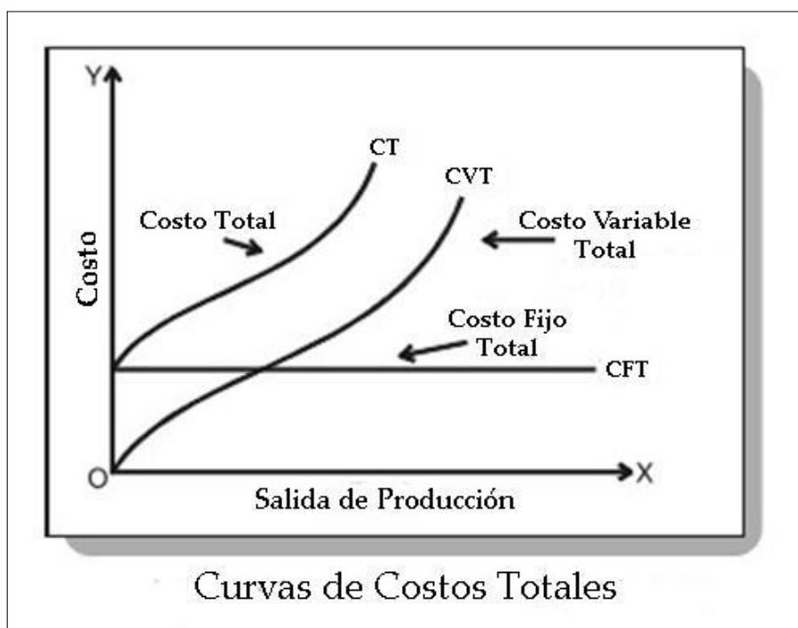
Figura 1. Grafico de Costo Total, Costo fijo y Costo Variable
